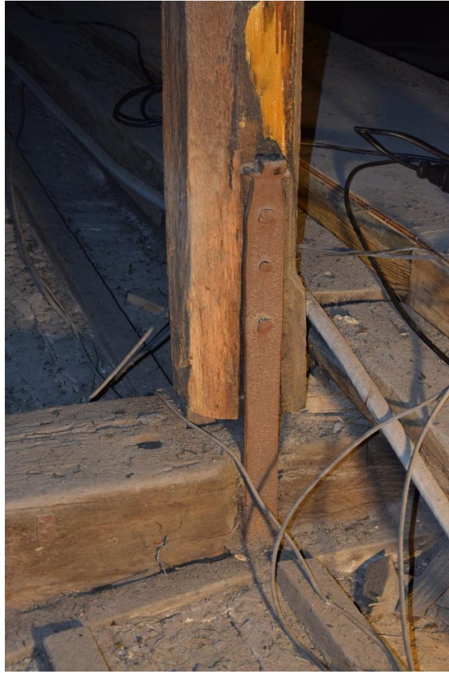
Figure 85. Huy, Église Saint-Mengold , assemblage du poinçon à l'entrait, détail d'un étrier (© Gabriel Bister, 2025).
