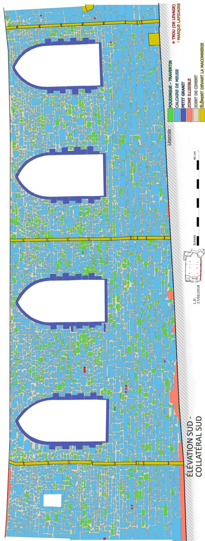
Figure 58. Huy, Église Saint-Mengold , le mur gouttereau sud (© Laetitia Demoulin [relevé pierre-à-pierre], 2018).
