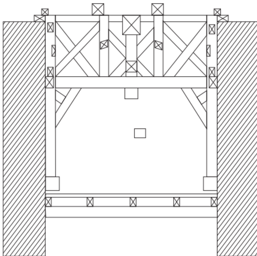
Figure 35. Huy, Église Saint-Mengold , coupe transversale de la charpente de la flèche jusqu'au premier niveau d'enrayure (© Gabriel Bister [Relevé et DAO], 2025).
