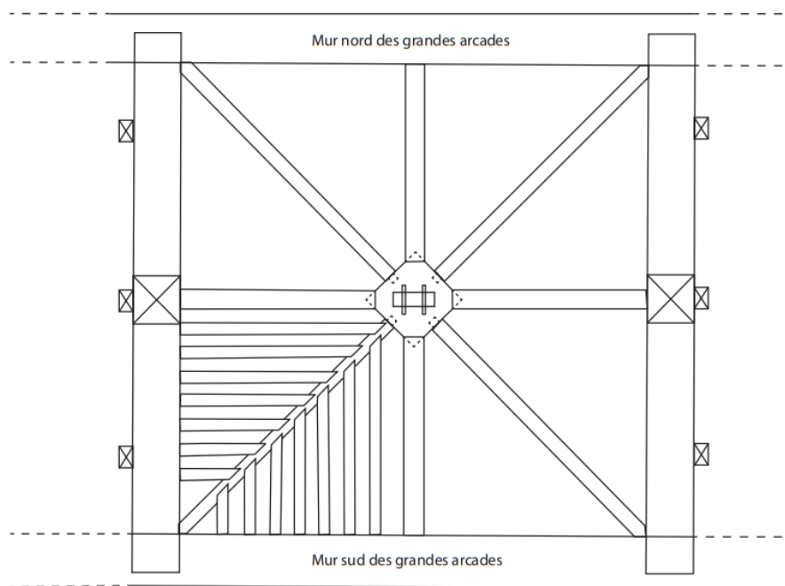
Figure 96. Huy, Église Saint-Mengold , plan d'une travée de la fausse-voûte en lattes et plâtre du XVIII e siècle, avec les entrails et poinçons (© Gabriel Bister, 2025).
