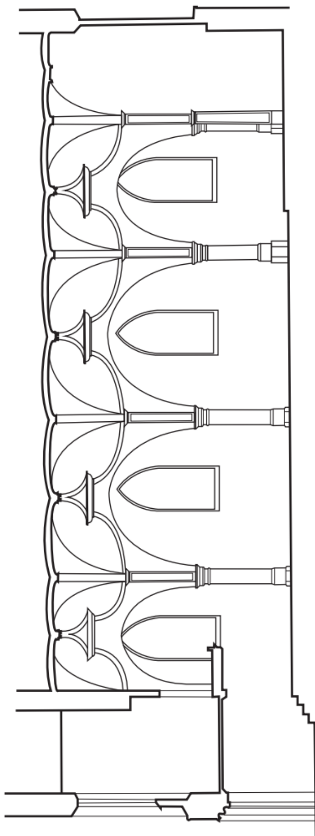
Figure 3. Huy, Église Saint-Mengold , coupe longitudinale de la nef. État en 1981 (© Guy Ciplet [relevé métrique] ; Gabriel Bister [DAO], 2025).
