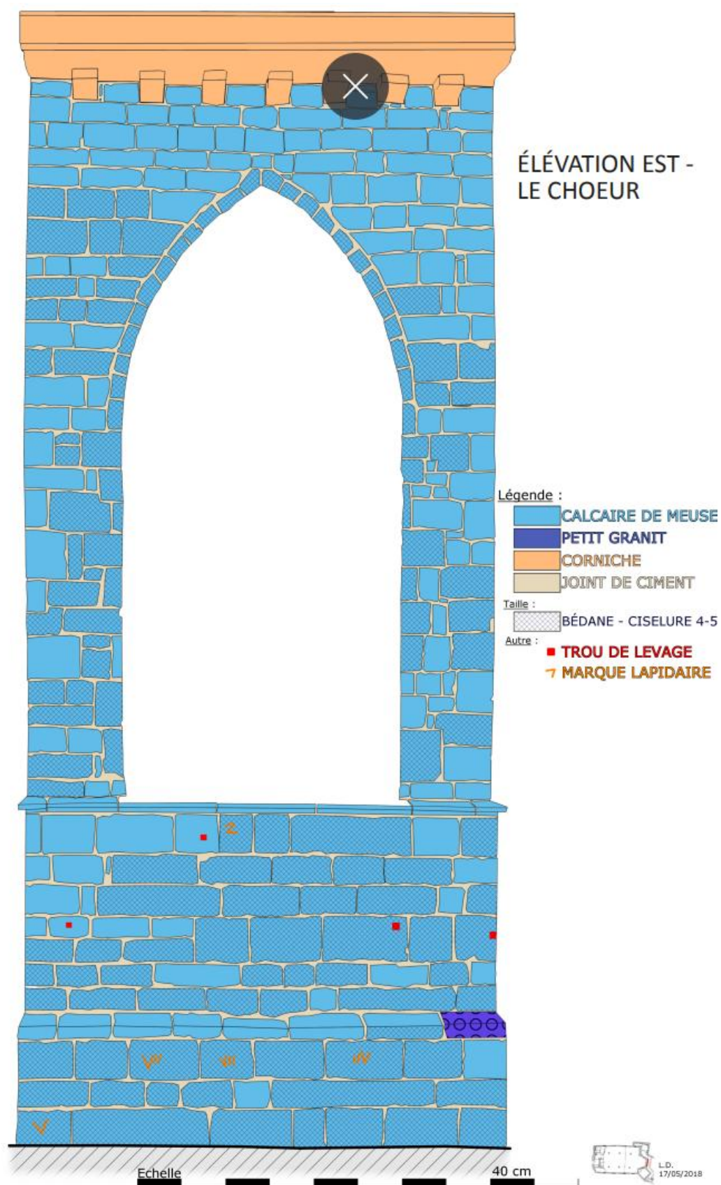
Figure 116. Huy, Église Saint-Mengold , le pan central du chevet (© Laetitia Demoulin [relevé pierre-à-pierre], 2018).
