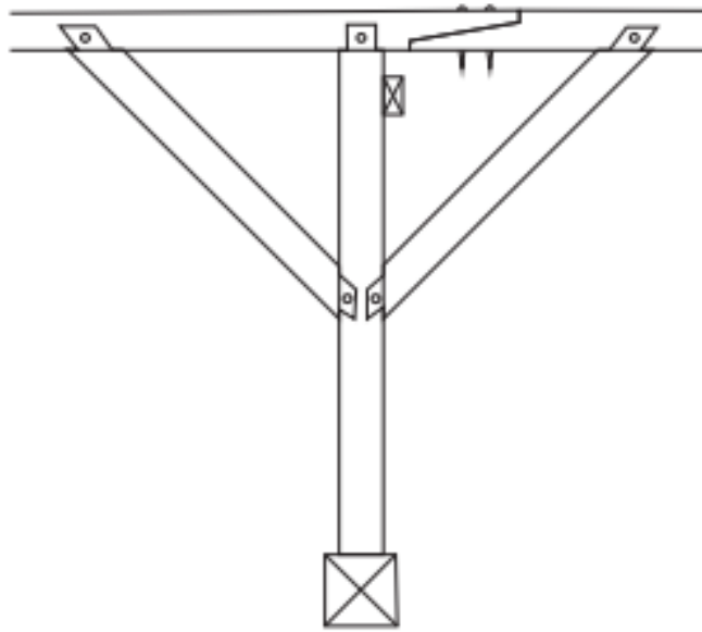
Figure 91. Huy, Église Saint-Mengold , croquis d'une potence (© Gabriel Bister, 2025).
