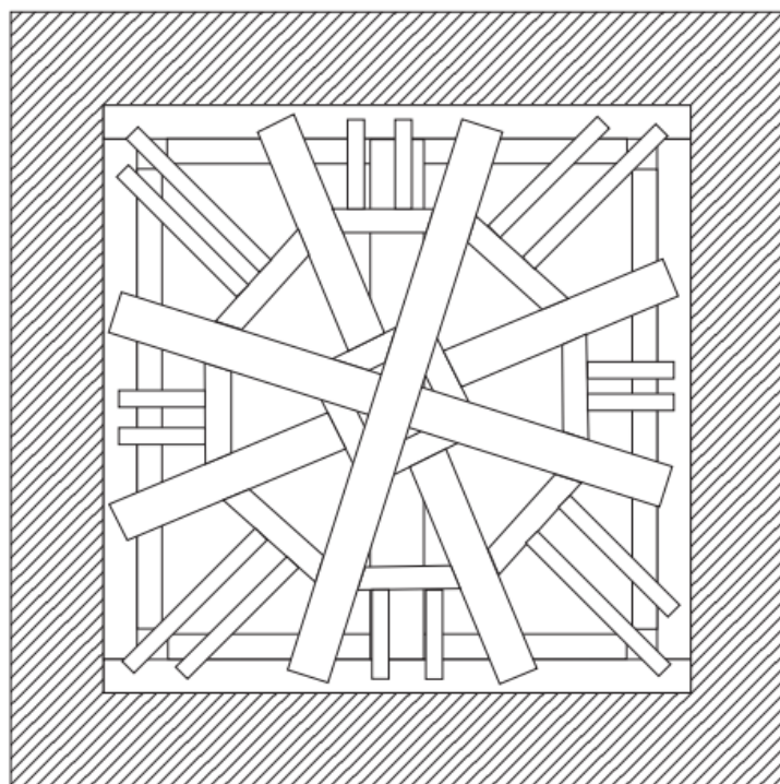
Figure 38. Huy, Église Saint-Mengold , plan du premier niveau d'enrayure de la charpente de la flèche (© Gabriel Bister [Relevé et DAO], 2025).
