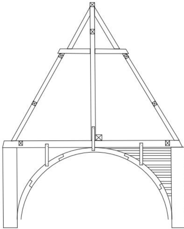
Figure 98. Huy, Église Saint-Mengold , coupe transversale de la fausse-voute en lattis et plâtre du XVIII e siècle, avec les arcs doubleaux (© Gabriel Bister, 2025).
