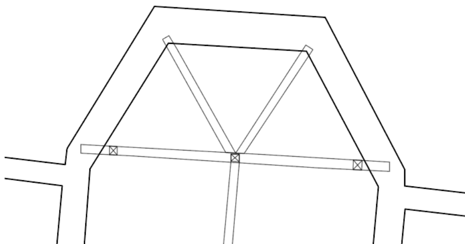
Figure 122. Huy, Église Saint-Mengold , plan de la charpente du chœur (© Guy Cipllet [relevé métrique] ; Gabriel Bister [DAO], 2025).
