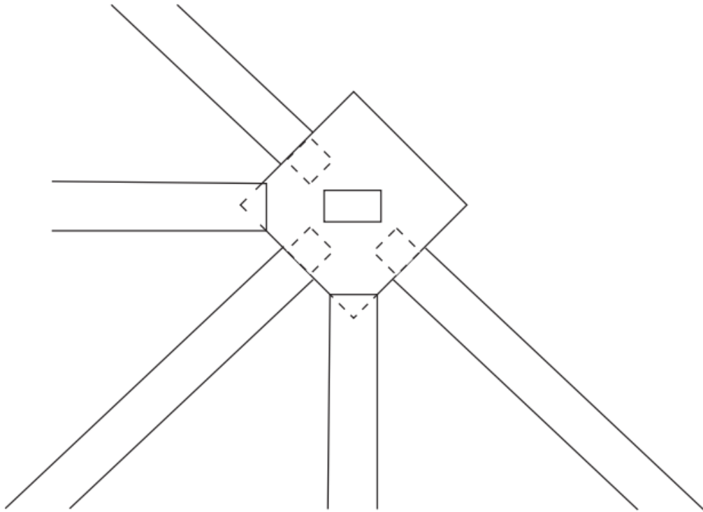
Figure 104. Huy, Église Saint-Mengold , détail de tirants de la fausse-voûte (© Gabriel Bister, 2025).
