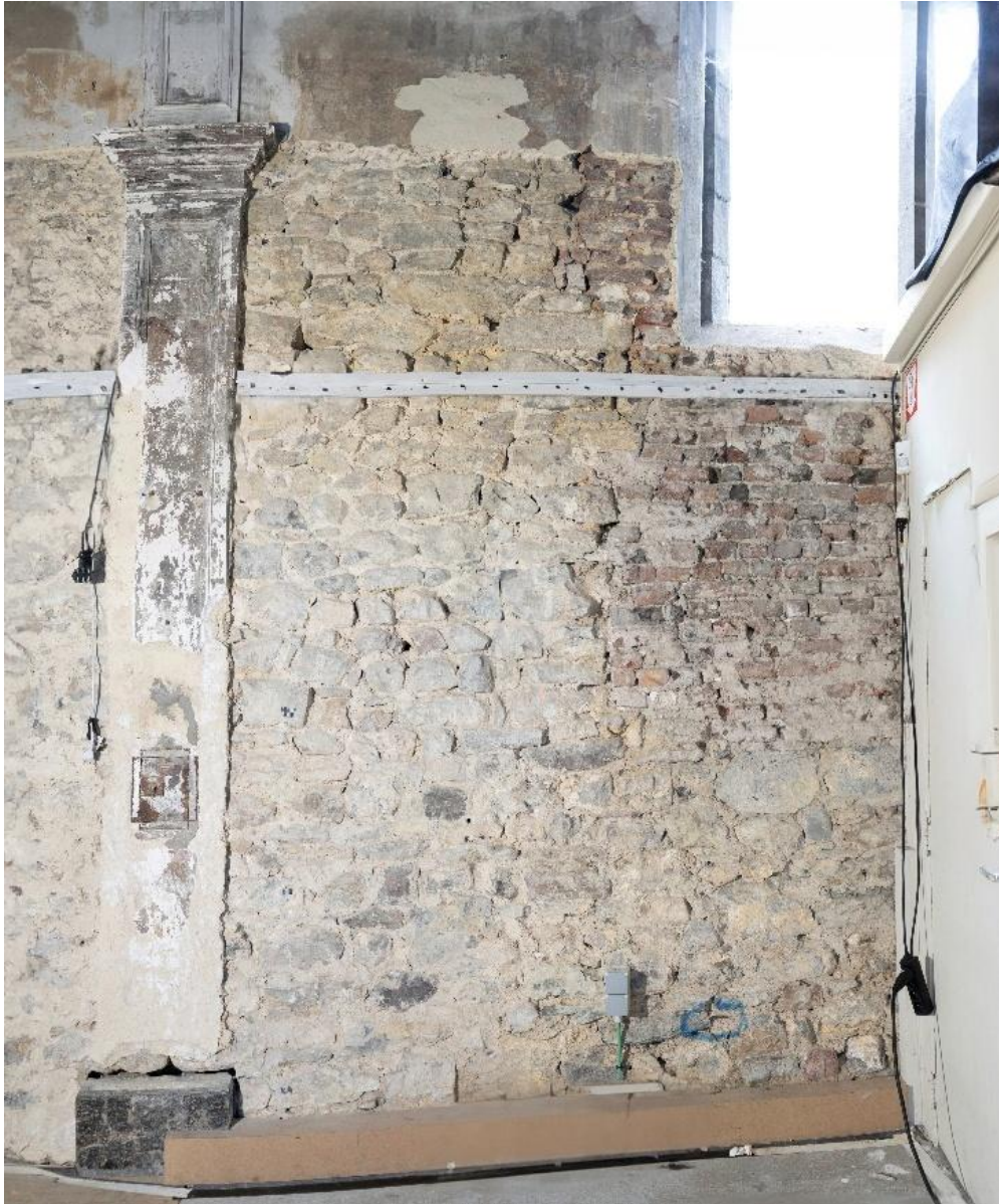
Figure 75. Huy, Église Saint-Mengold , le mur gouttereau du collatéral sud à hauteur de la première travée : vue depuis la nef (© Alexandre Bister [relevé photographique et orthophotographie], 2025).
