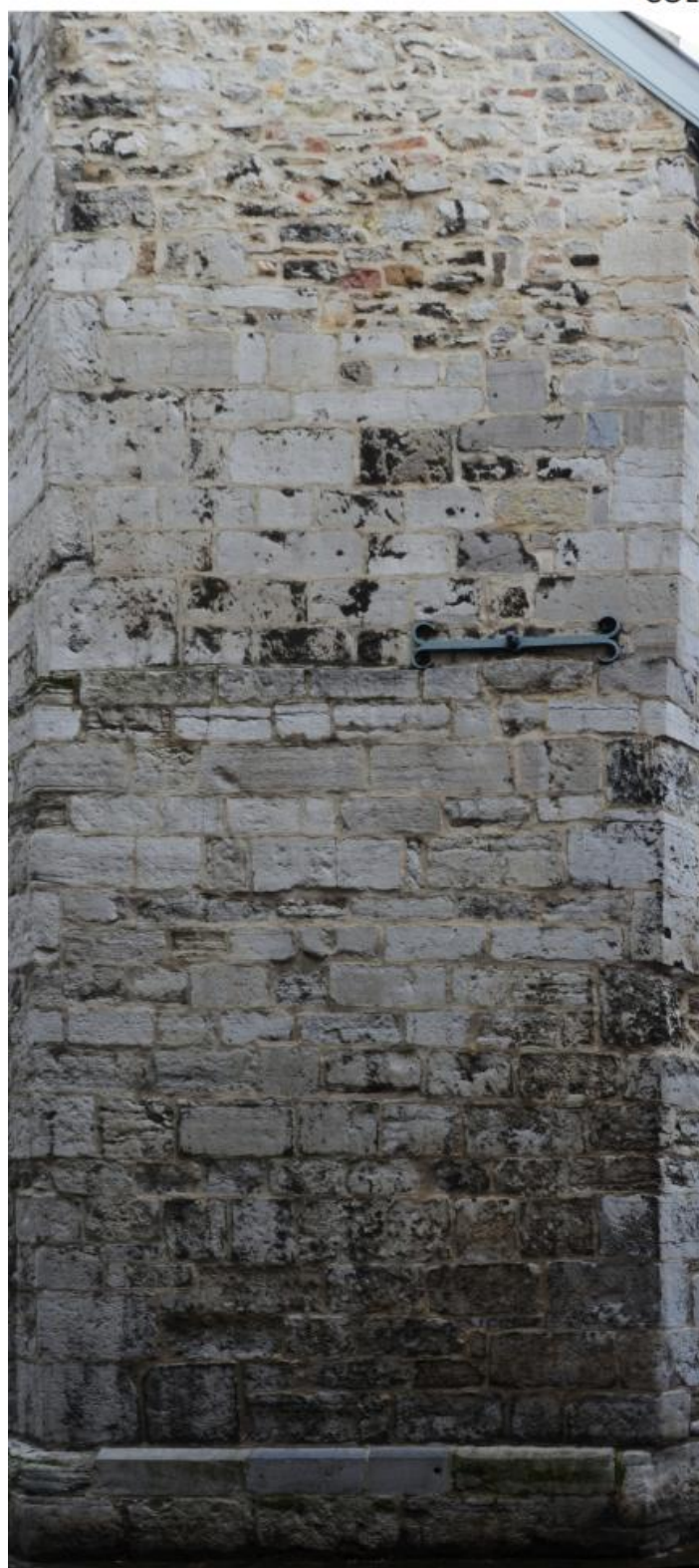
Figure 54. Huy, Église Saint-Mengold , façade occidentale du collatéral sud (© Lactitia Demoulin[relevé photographique et orthophotographie], 2018).
