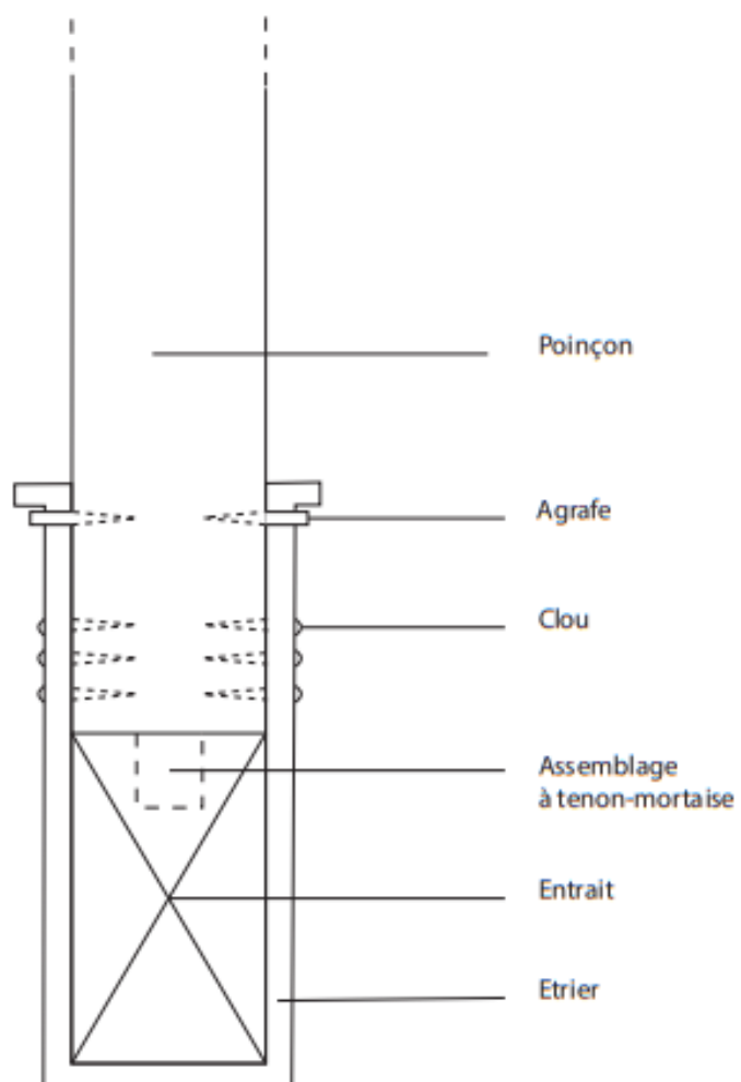
Figure 87. Huy, Église Saint-Mengold , croquis de l'assemblage d'un poinçon à l'entrait avec étrier (© Gabriel Bister, 2025).
