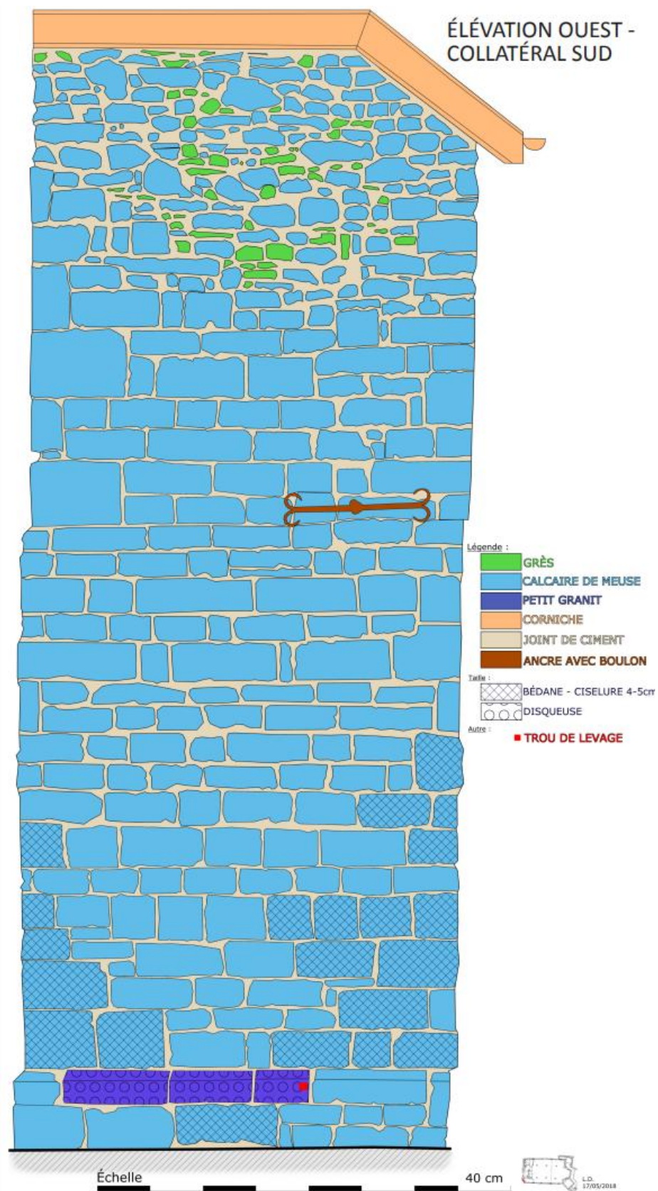
Figure 55. Huy, Église Saint-Mengold , façade occidentale du collatéral sud (© Laetitia Demoulin [relevé pierre-à-pierre], 2018).
