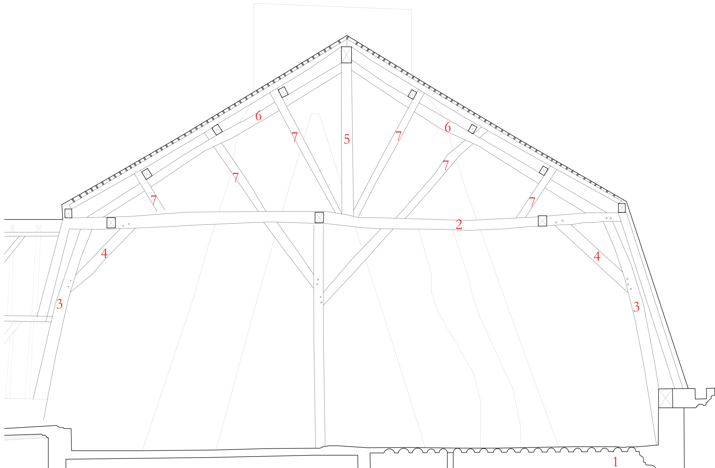
Le château de Warelles Charpente du corps de logis principal - A la Mansart Pauline Ducci
