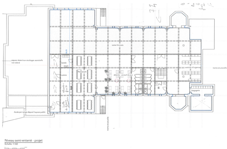
Figure 23 – Plan R-1 du projet de l'église diocésaine Notre-Dame des Victoires à Lille - Atelier Sébastien Muteba Architecture + design
