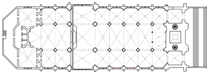
Figure 50 – Plan de l'église néogothique de 1865 – Production personnelle
