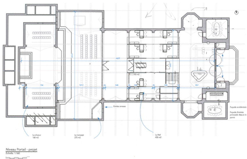
Figure 22 – Plan RDC du projet de l'église diocésaine Notre-Dame des Victoires à Lille - Atelier Sébastien Muteba Architecture + design
