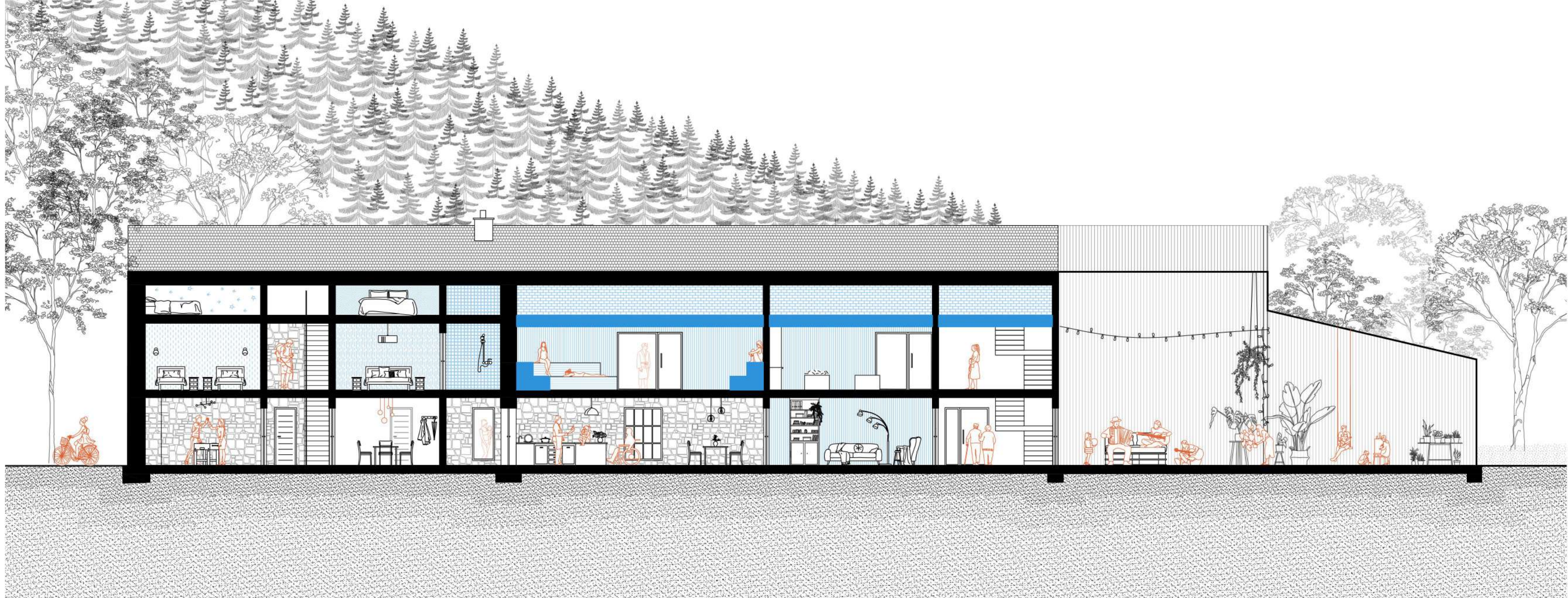
Coupe longitudinale A-A'
