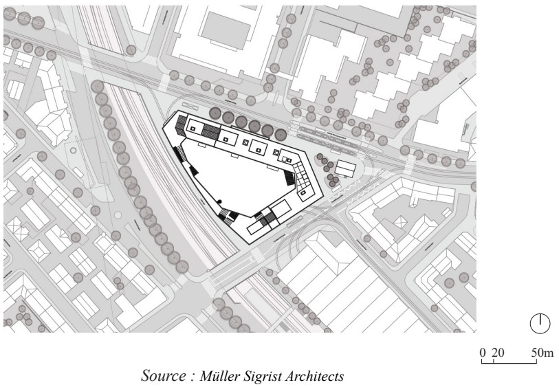
Fig. 27: Plan de situation
