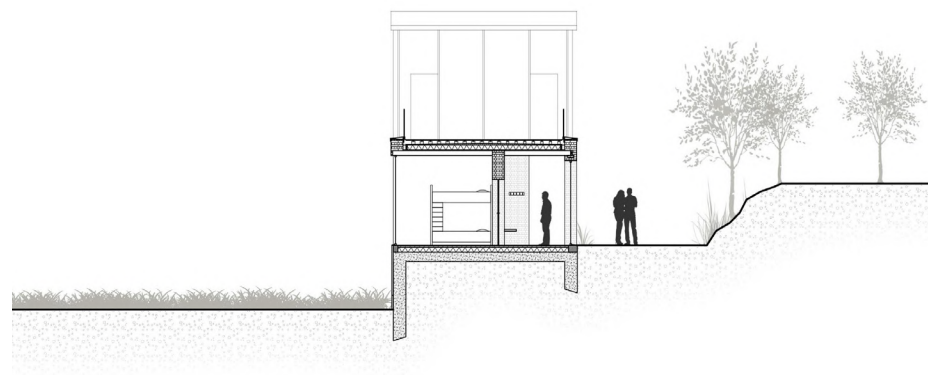
Coupe transversale du projet et du chemin, encadrés d'un côté par le champ et de l'autre par la végétation. Document réalisé par l'auteur.
