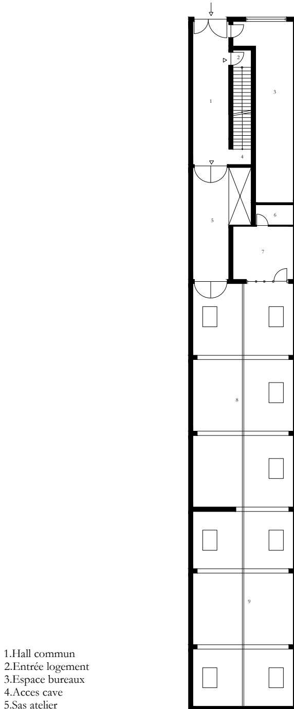
Figure 103 : Plan d'un atelier de menuiserie
