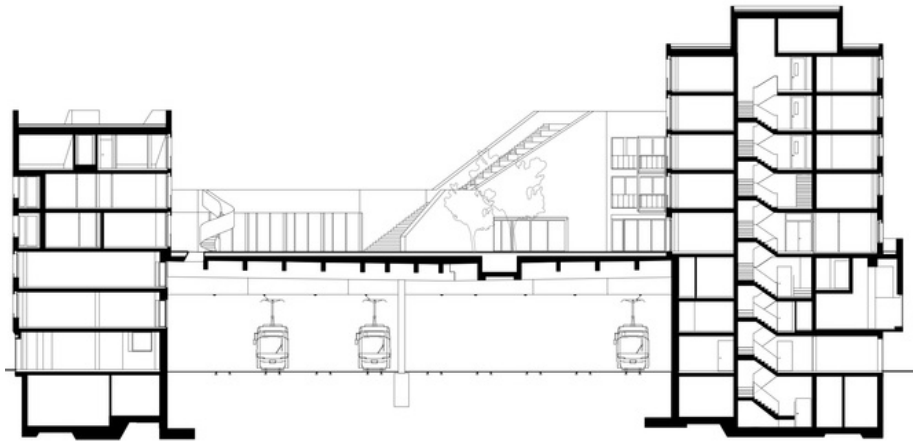
Figure 13: Coupe longitudinale, Kalkbreite
