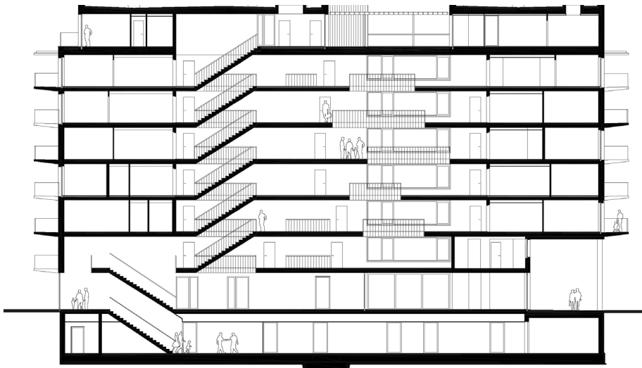
Figure 10: Coupe longitudinale, Woonprojekt Wien
