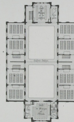
PLAN DE L'ÉTAGE (B TE PRINCIPAL)
