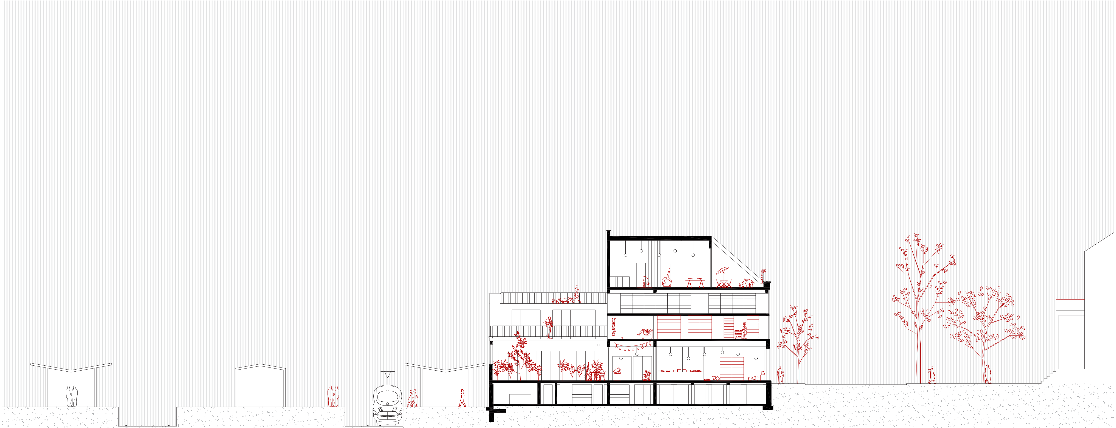
Coupe A-A'
