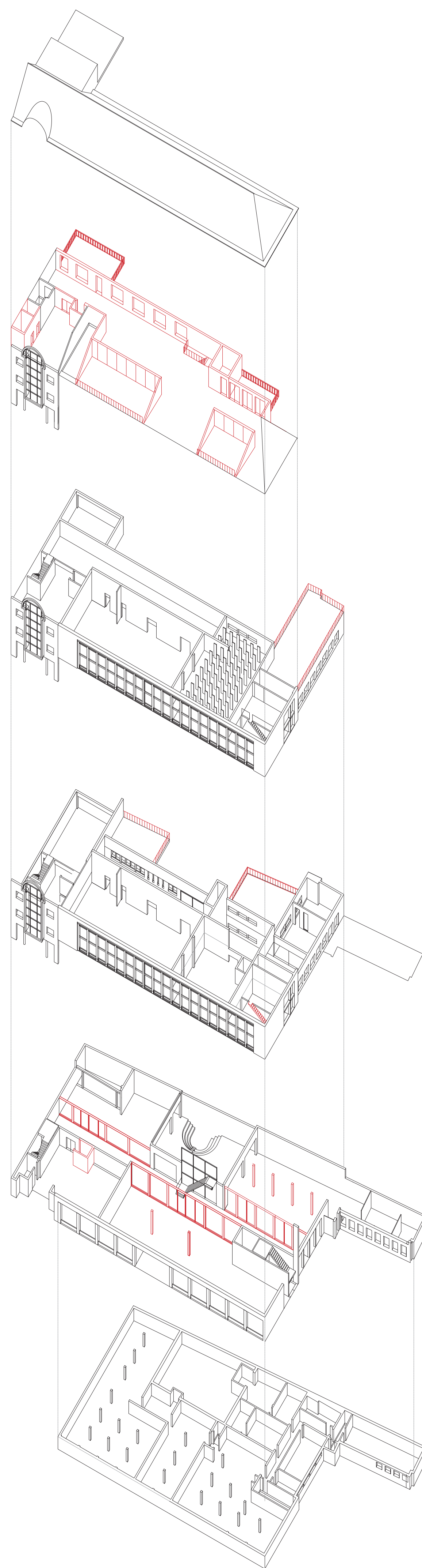
Situation projetée
