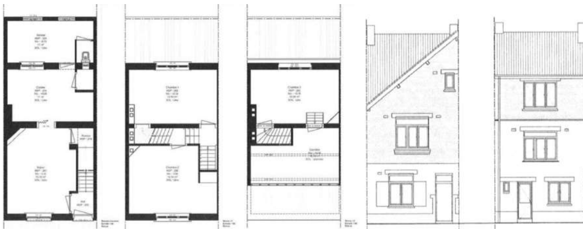
Figure 99 : Annexe - plans et élévations d'une maison à deux mitoyens avec entrée à rue et simple galbe (Foyer Anderlechtois, s.d.).
