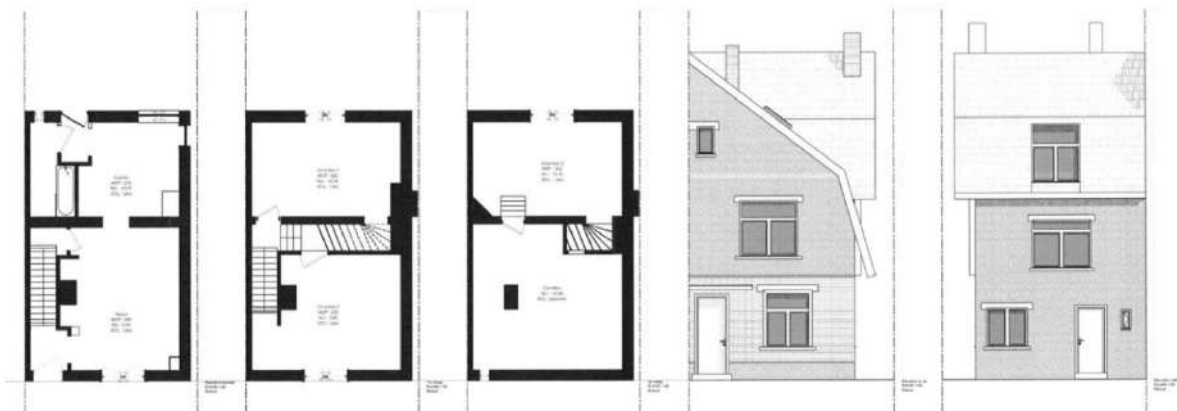
Figure 98 : Annexe - plans et élévations d'une maison à deux mitoyens à demi-galbe (Foyer Anderlechtois, s.d.).
