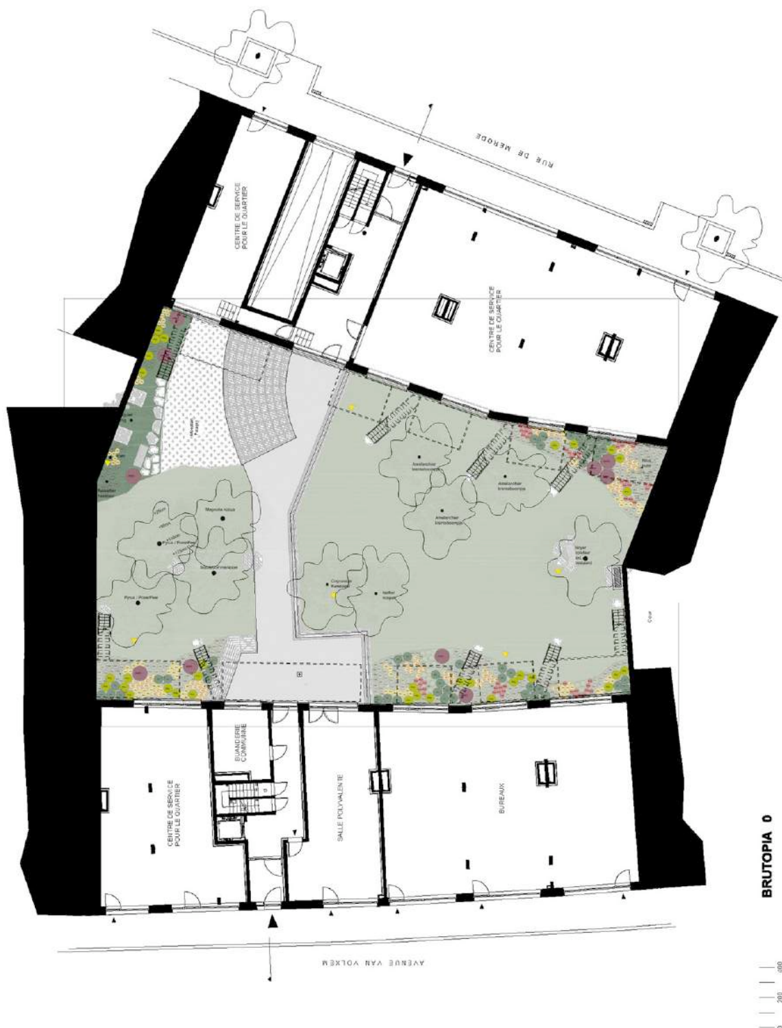
Figure 100 : Annexe - plan RDC de Brutopia (Stekke + Fraas architecte(s)(n), s.d.).
