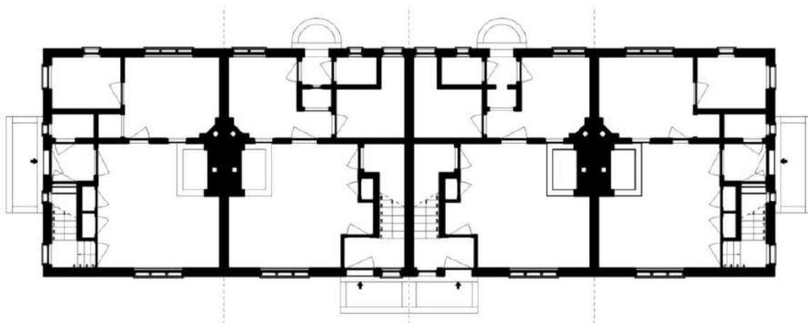
Figure 96 : Annexe - plans d'un groupement d'habitation d'un îlot dit "expérimental" (Foyer Anderlechtois, s.d.).
