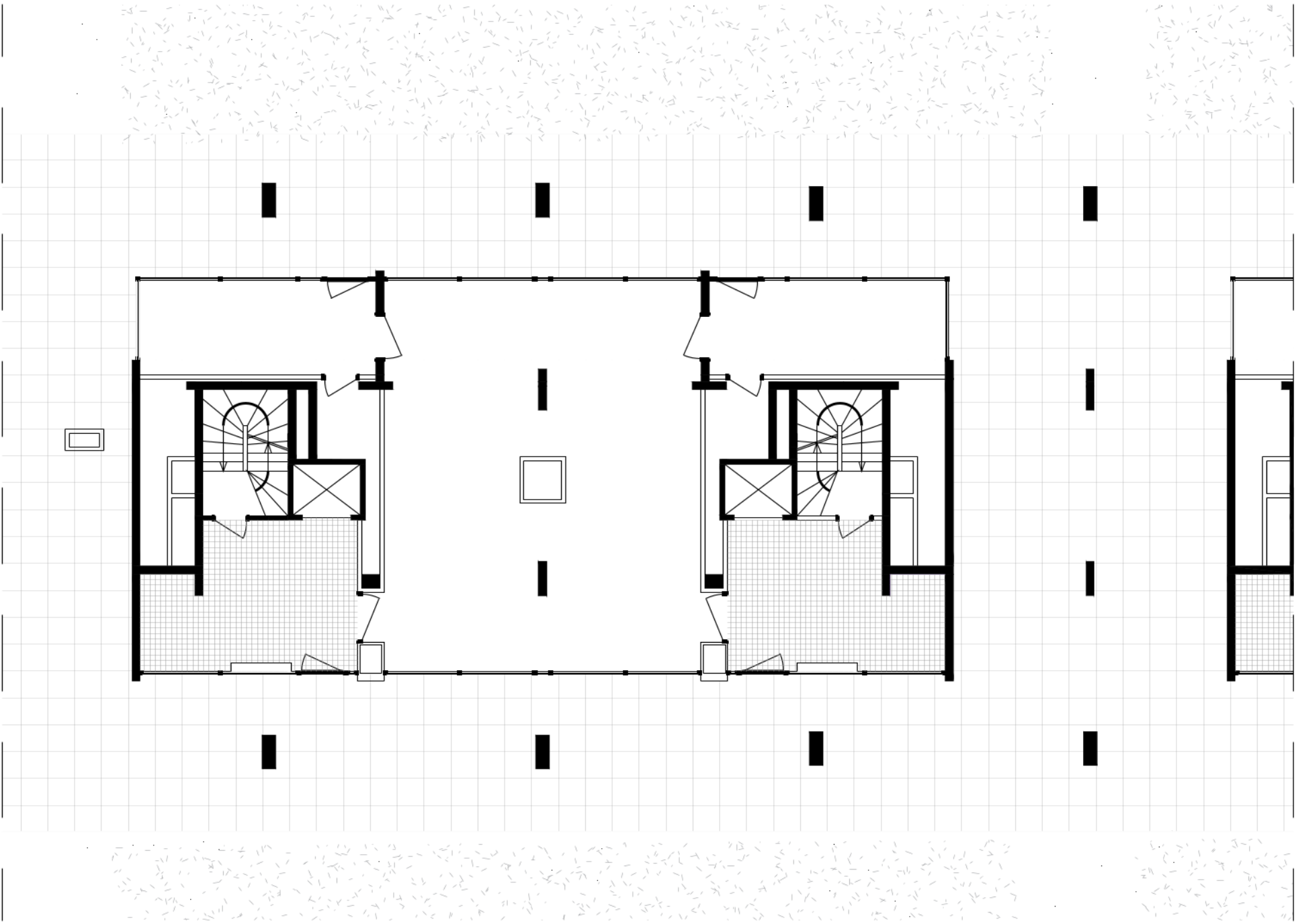
Bloc 4 : Plan de situation existante
