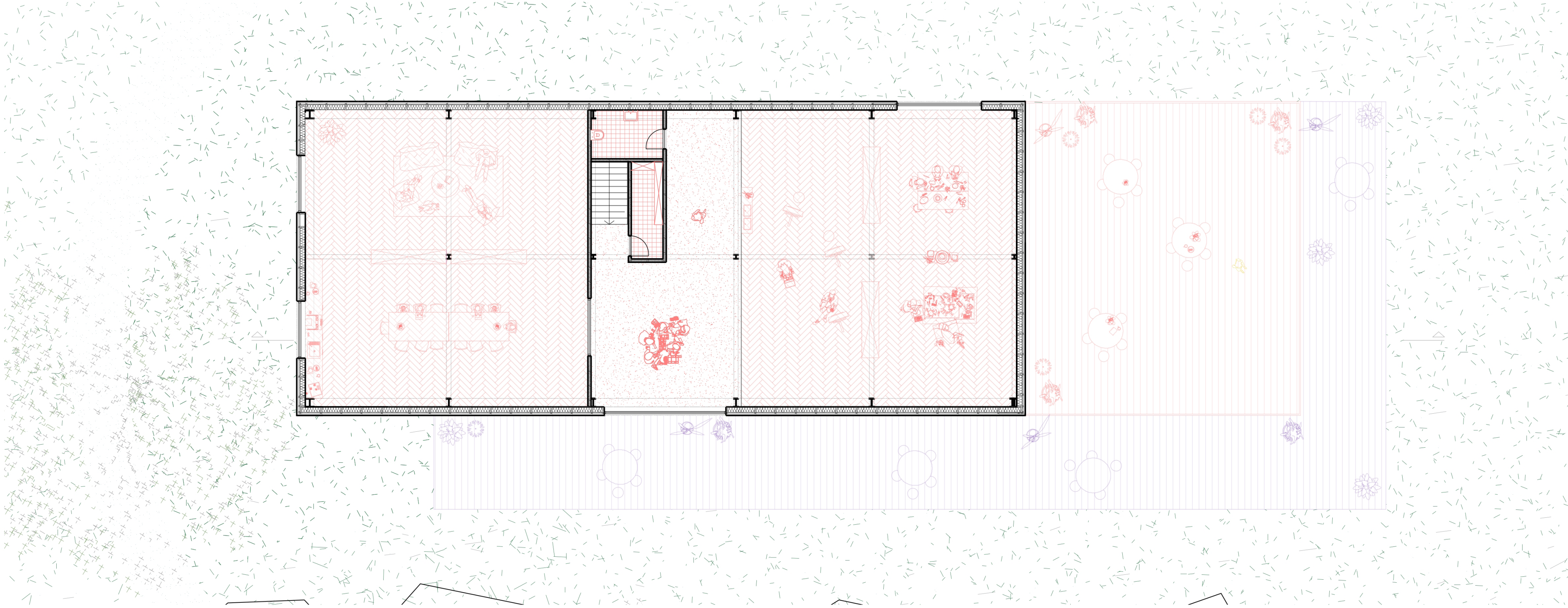
Plan espace pour filles ( mezzanine )
