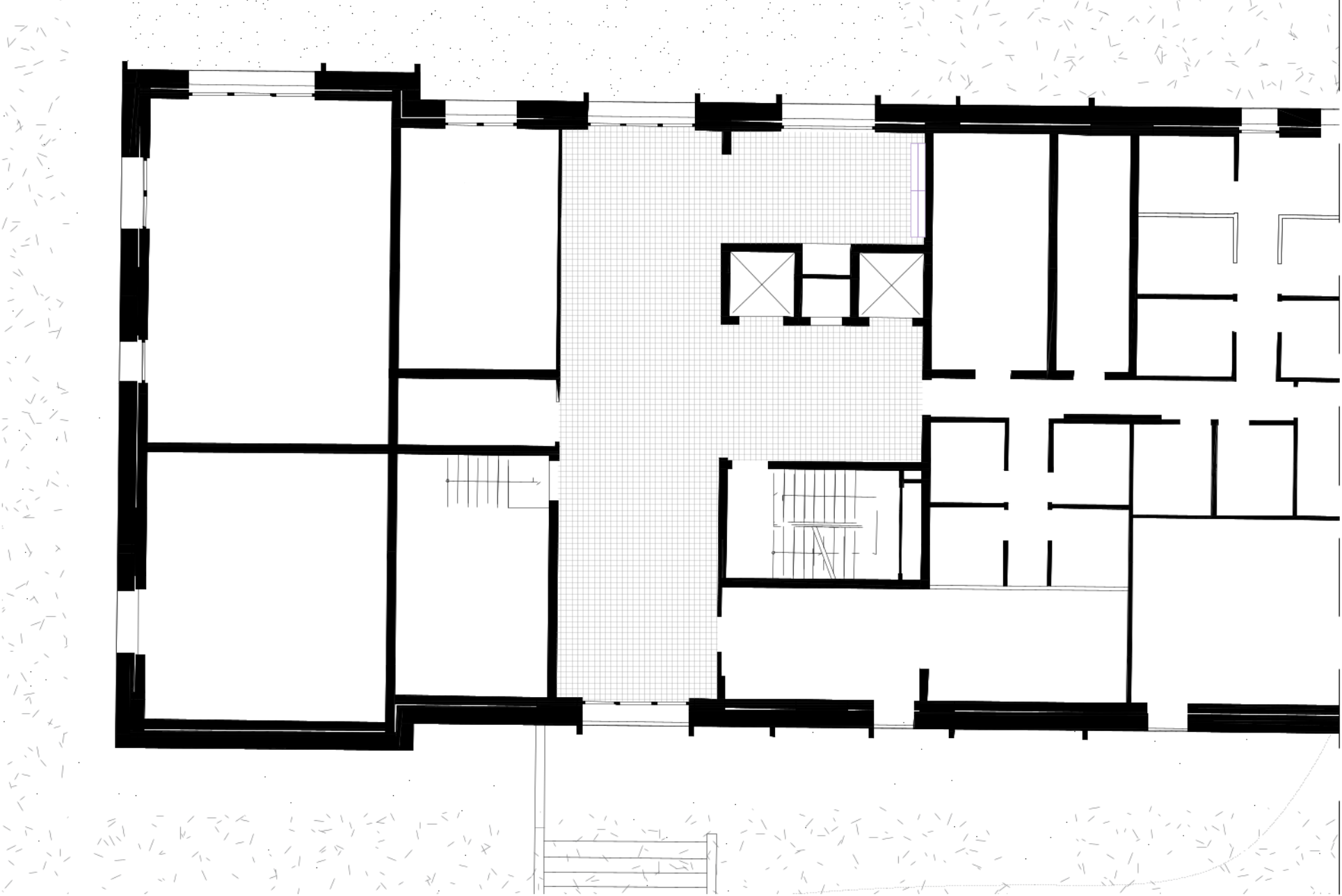
Bloc 10 : Plan de situation existante
