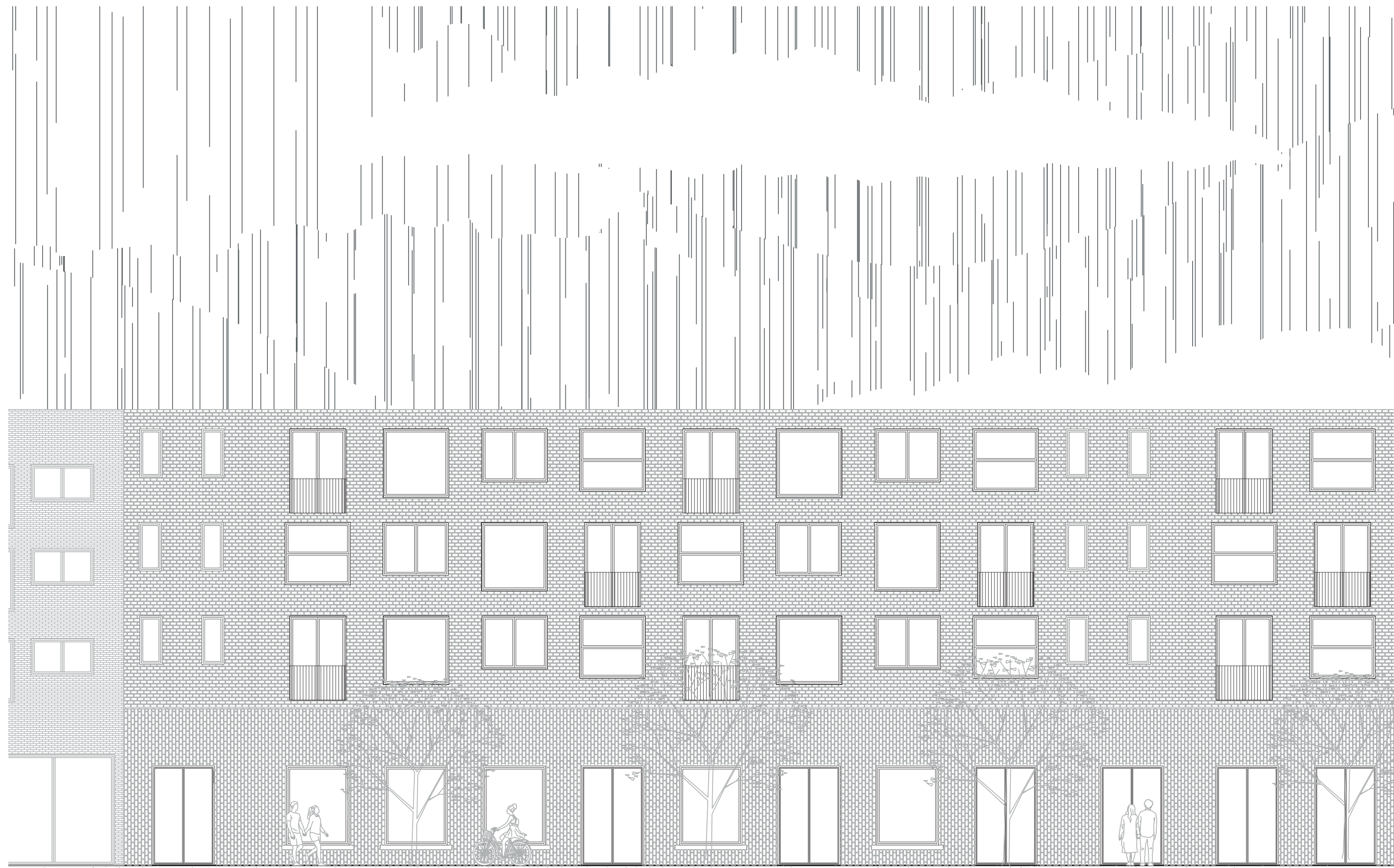
Elévation Sud
