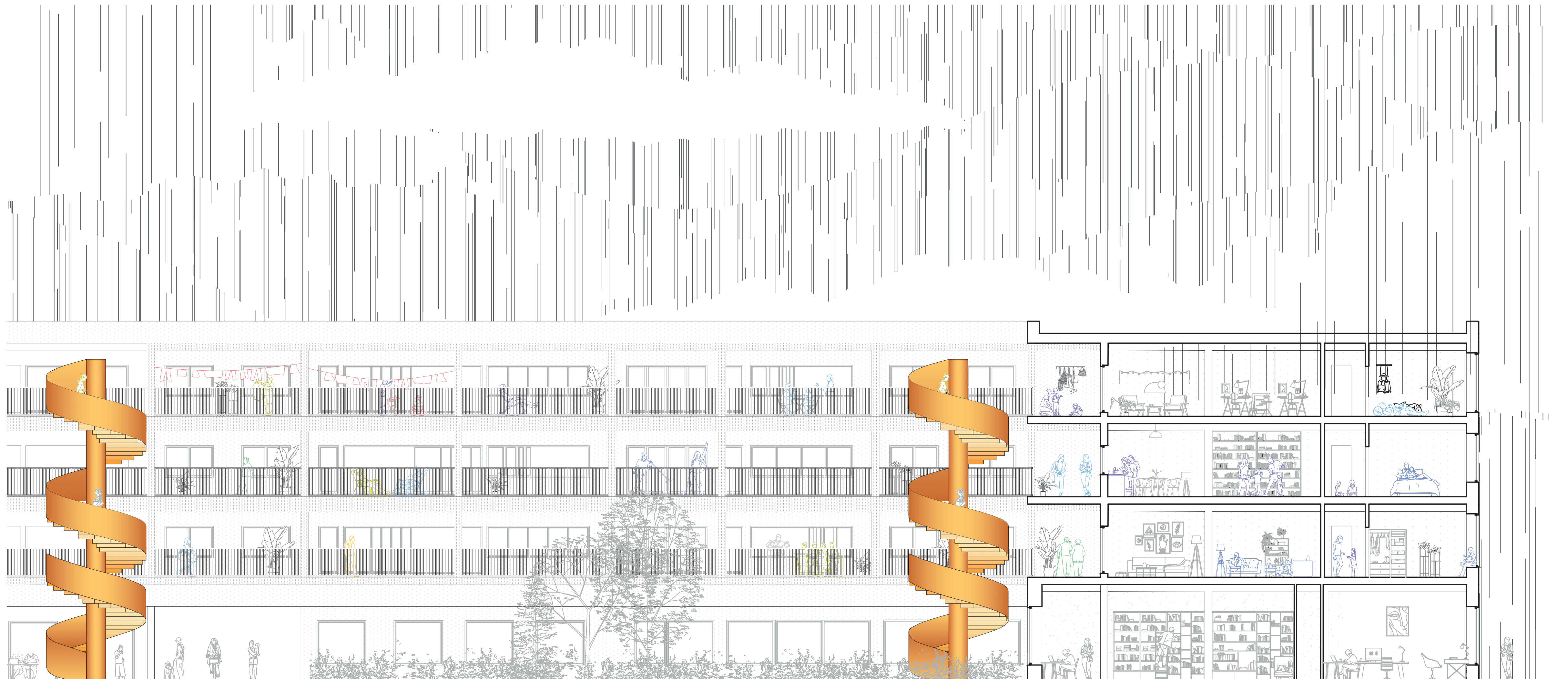
Elévation / Coupe Nord
